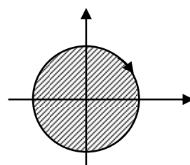
|z| > R
