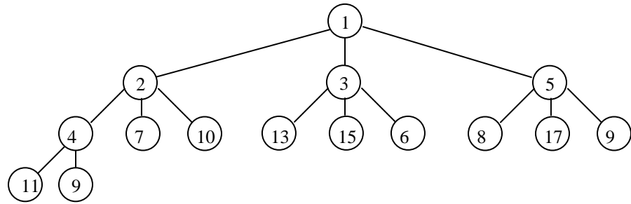
Hình 11.3 . d-heap
